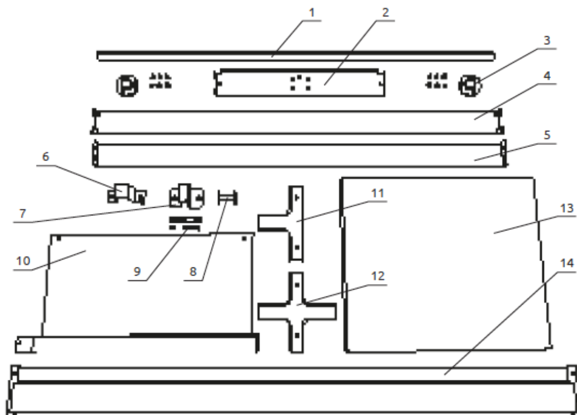
Рис. 1а. Дополнительные элементы стеллажа ТСУ.
