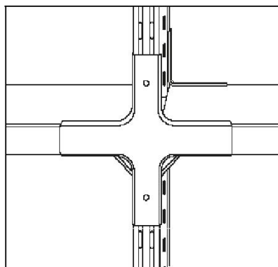
Рис. 15. Установка крестовины.
