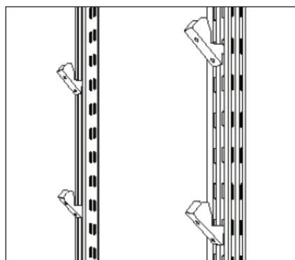
Рис. 8. Установка кронштейнов.
