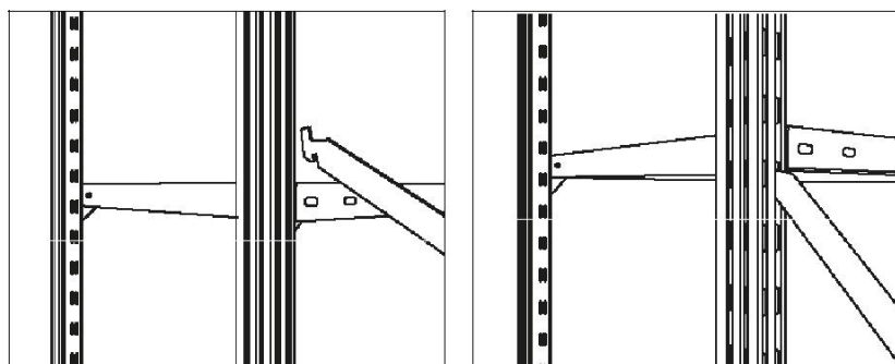
Рис. 10. Установка растяжки крестовины жесткости в стойку.
