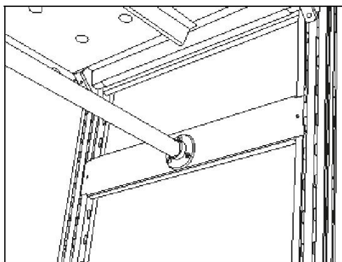
Рис. 17. Установка штанги.
