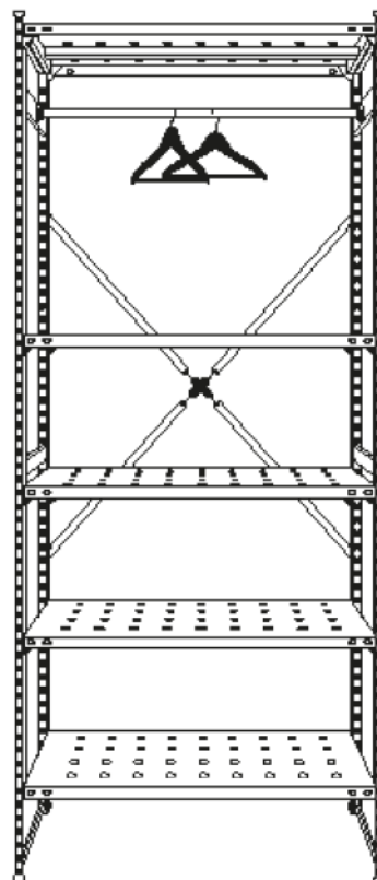
Рис. 13. Стеллаж ТСУ со штангами для одежды.
