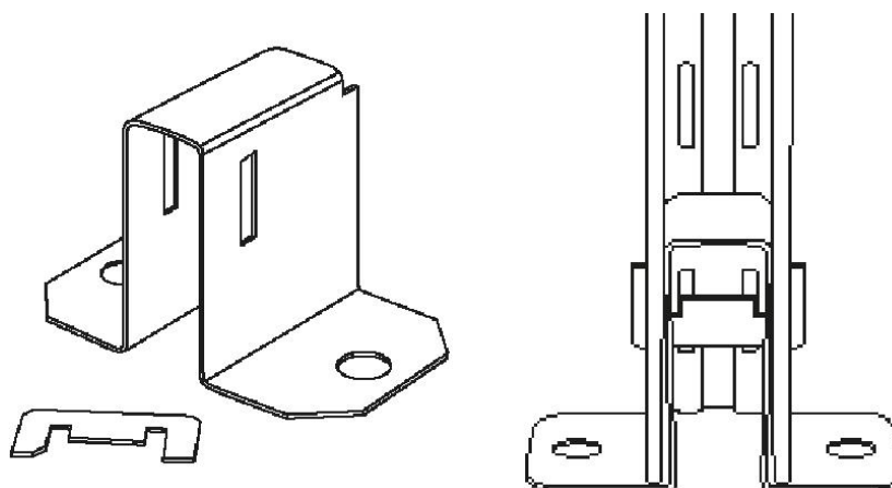
Рис. 22. Подпятник.
