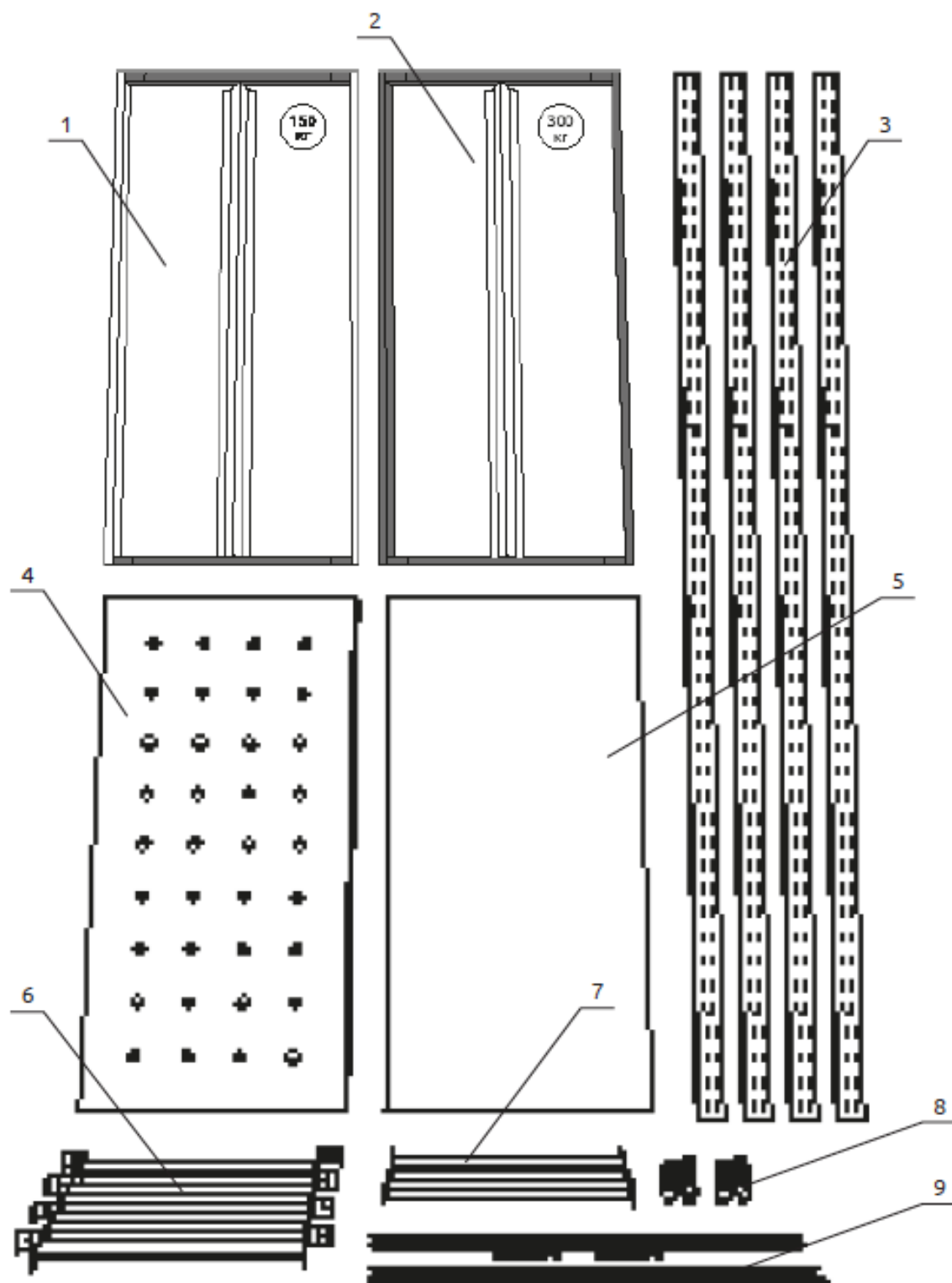
Рис. 1. Комплектация стеллажа.
